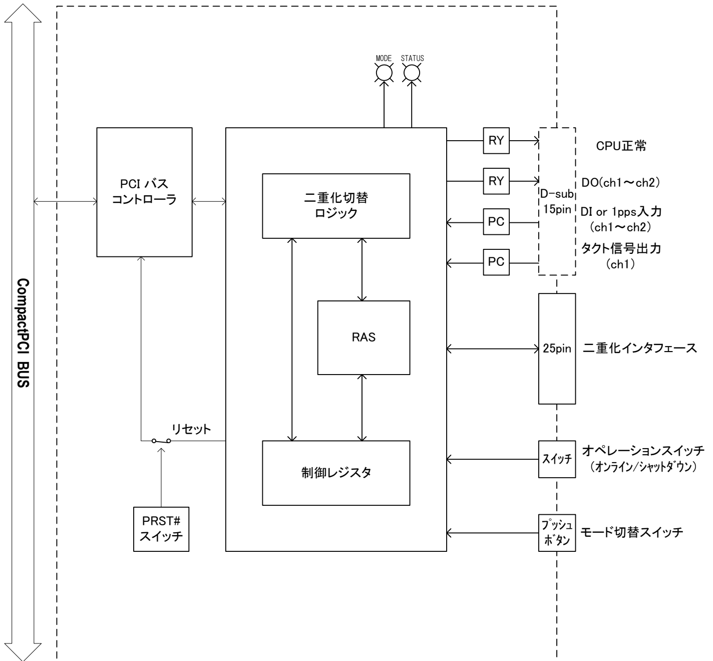
CPDIO03 ブロック図
